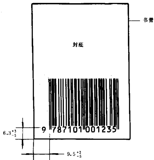
图 1 条码位于封底左下角， 条的方向与书脊平行
